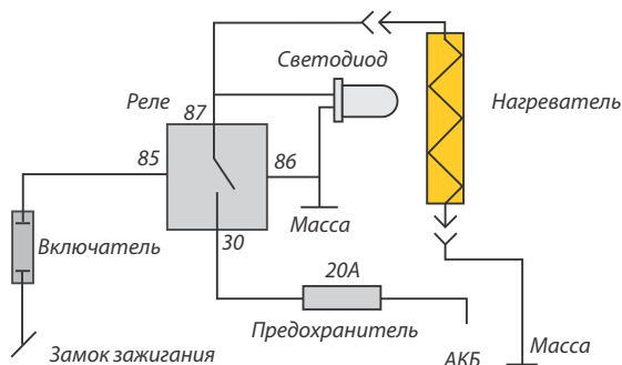
Схема подключения нагревателя к бортовой сети автомобиля.
